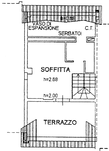
PIANO SECONDO (Soffitta)
